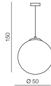
Sweet 50 AZ0443 E27 3x 60W acrylic metal/chrome
